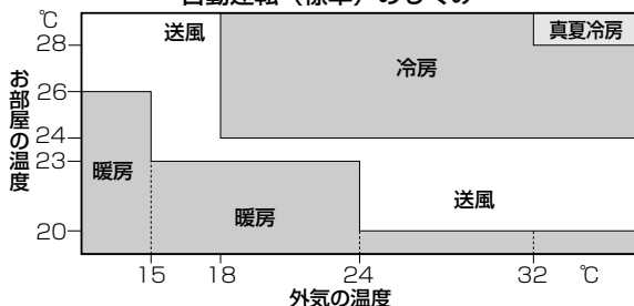
自動運転（標準）のしくみ
