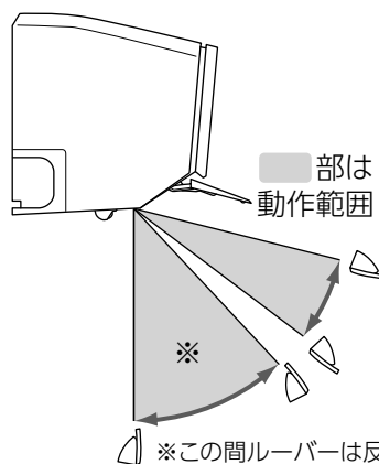
上下風向ルーバーの動作
