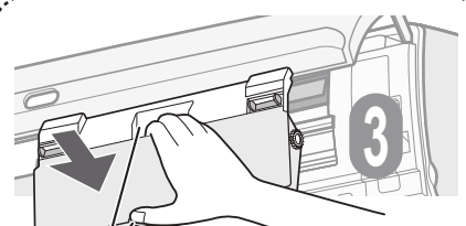
ダストボックスの持ち手
