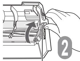
ブラシ押さえのつまみ(灰色)
