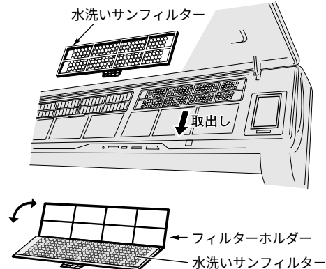
水洗いサンフィルター
