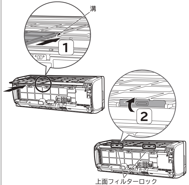
上面フィルターロック
