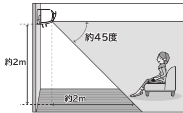
お部屋を横から見た場合
