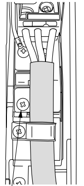
⑧ アースねじ アース端子を接続するときは端子台カバーを外して行います。
