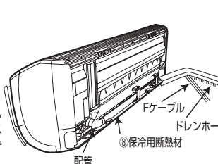
⑧保冷用断熱材 ⑨配管押さえ (配管押さえは、2カ所どちらでも取り付けられます。配管整形のよい所で固定してください。)
