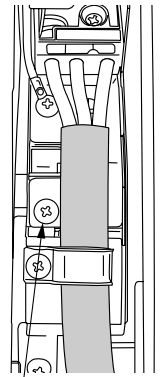
⑧アースねじ アース端子を接続するときは端子台カバーを外して行います。
