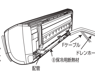
直引きの配管ドレンレイアウト
