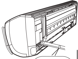
Fケーブル、配管、ドレンホースをテープ止めます。
