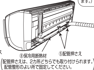
⑧保冷用断熱材 ⑤配管押さえ
