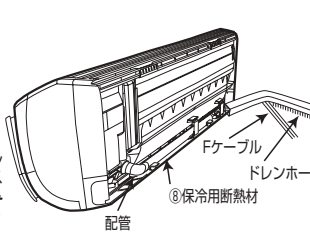
⑧ 保冷用断熱材 (配管押さえは、2カ所どちらでも取り付けられます。配管整形のよい所で固定してください。)
