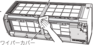
前面用ワイパーカバー
