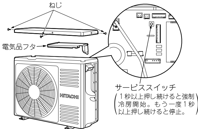
RAC-DT40W2、DT50W2
