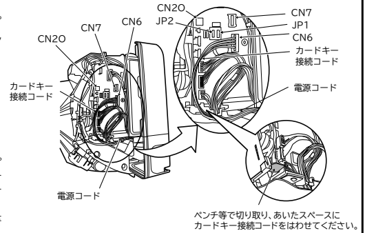
上図はカードキー(CN6)接続時 ペンチ等で切り取り、あいたスペースにカードキー接続コードをはわせてください。
