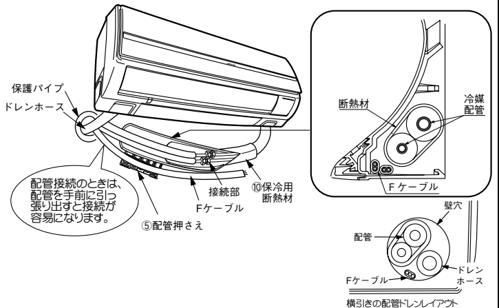
配管・ドレンホース・Fケーブルをまとめ、テープで仮止めます。
