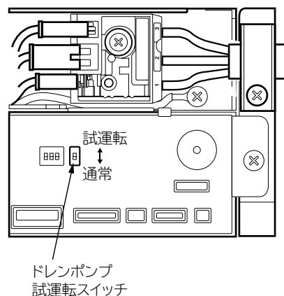
室内機電気品
