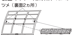
固定部（2カ所）
