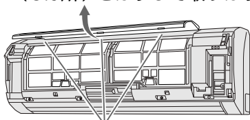
ツメ (3カ所)
