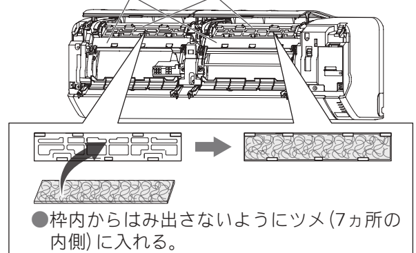
ダストボックス取付部
